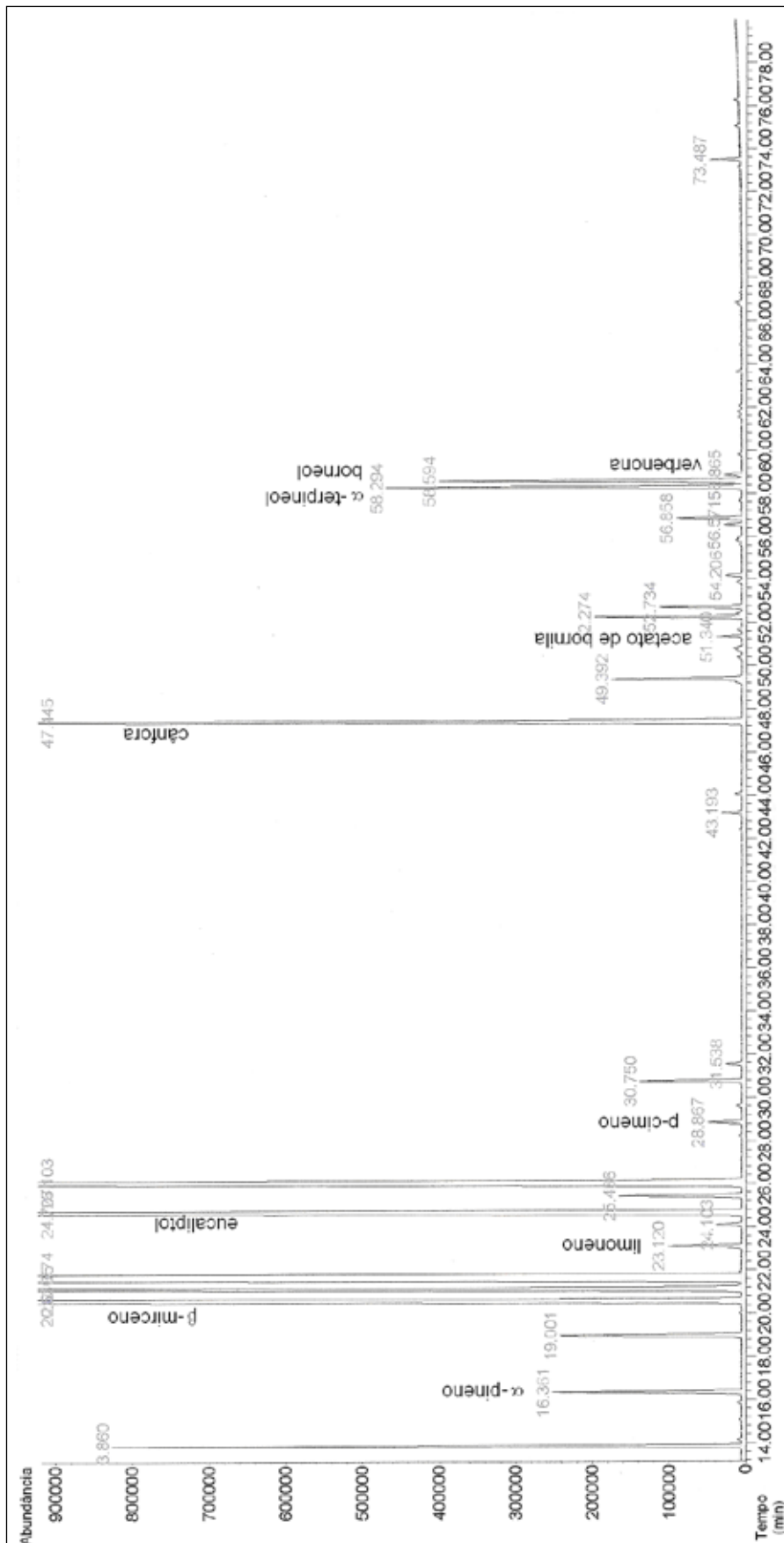
Figura 1 – Cromatograma ilustrativo obtido com o óleo volátil de Rosmarinus officinalis L por cromatografia gasosa acoplada a detector de massas.
